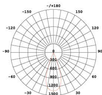
36° fascio/beam
