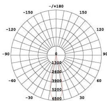
24° fascio/beam
